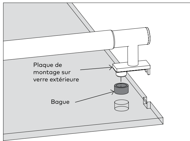
2.4.2 Placer la bague sur la plaque de montage extérieure en verre.
