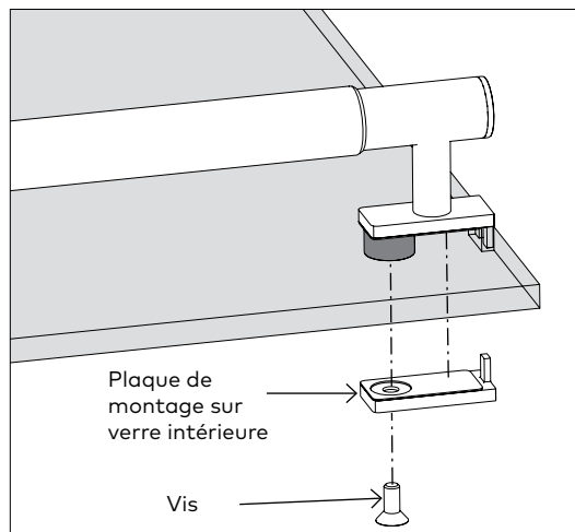
2.4.4 Fixer la plaque de montage sur verre intérieure (à travers le verre) à la poignée extérieure avec la vis incluse de 5/16 po-18 x 3/4 po.
