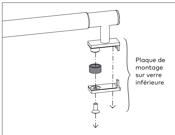
2.4.1 Démontez la plaque de montage sur verre inférieure.
