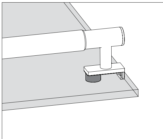
2.4.3 Placer la poignée extérieure contre le verre.
